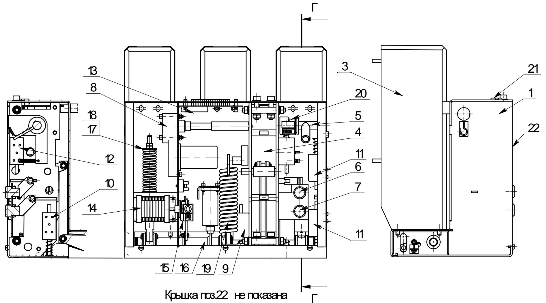
Общий вид выключателя.Рис.1
